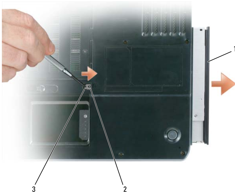
1 광학 드라이브 2 광학 드라이브 보호 나사 3 노치
